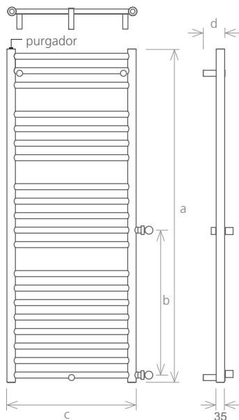
BL1400 IO (in&out) - Ligações laterais
