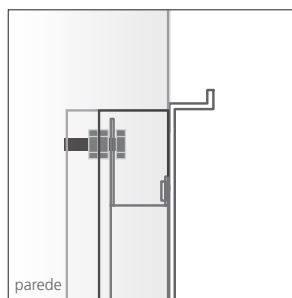
VISTA LATERAL
